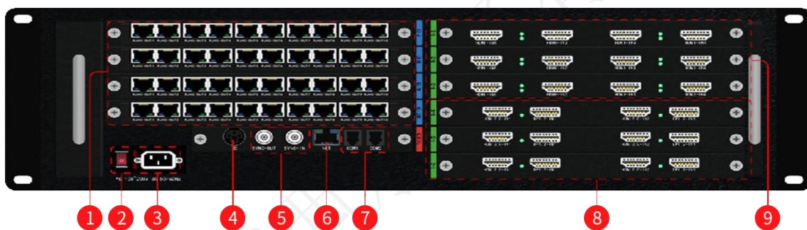
后面板
