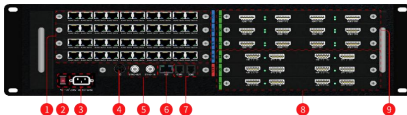
后面板
