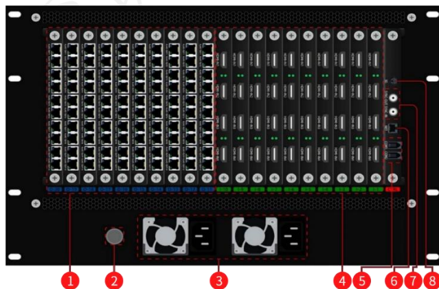
后面板
