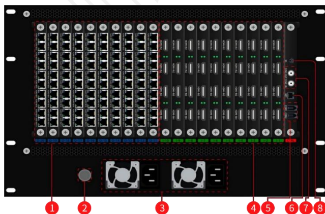
后面板
