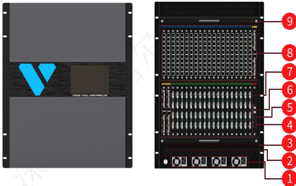
前面板
