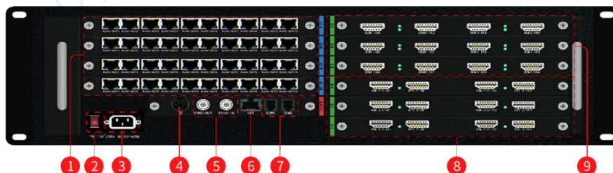
后面板
