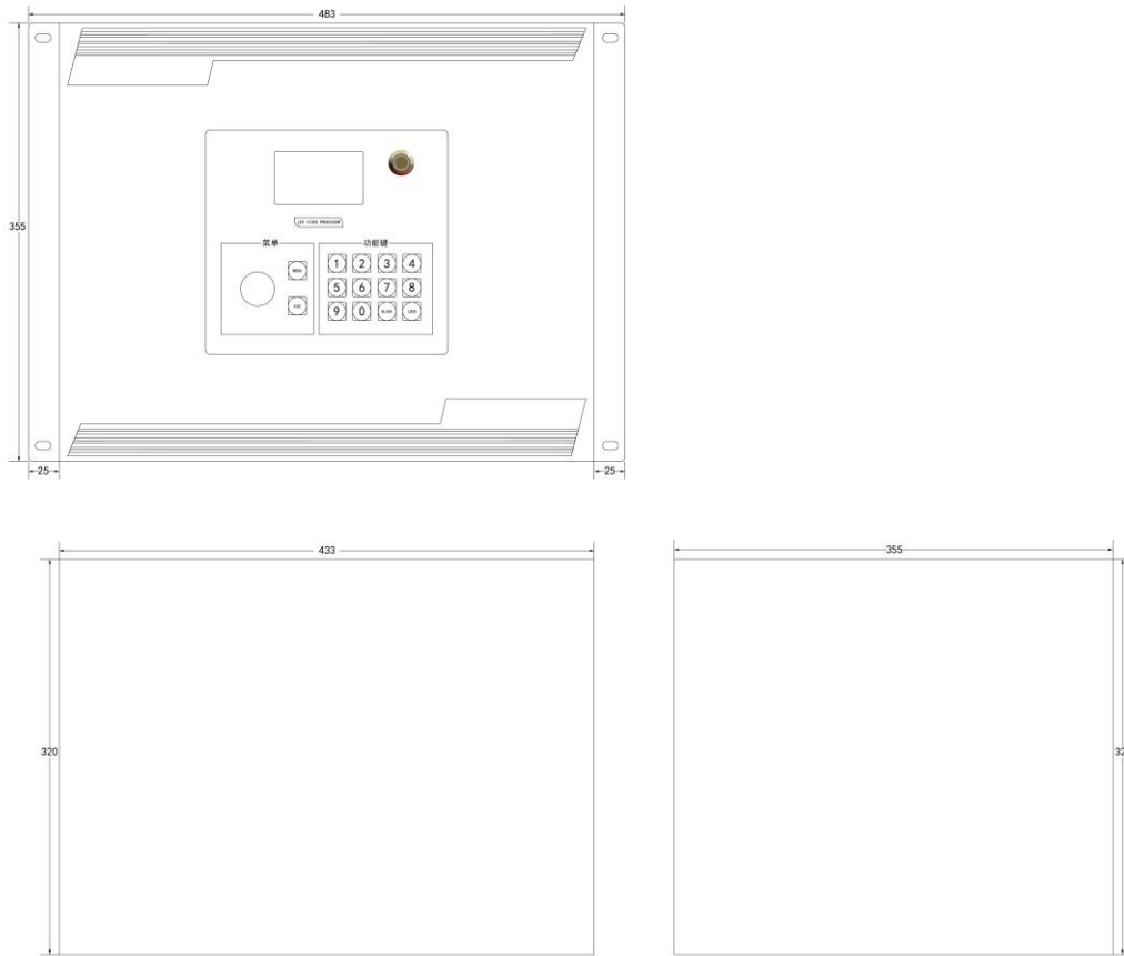
8U 尺寸图
