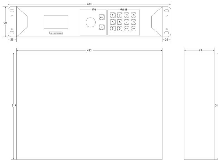
2U 尺寸图
