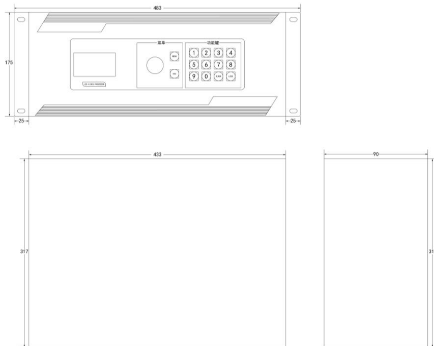
4U 尺寸图
