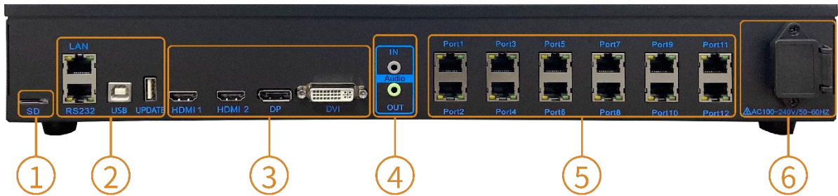
后面板
