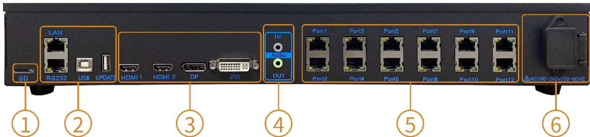
后面板
