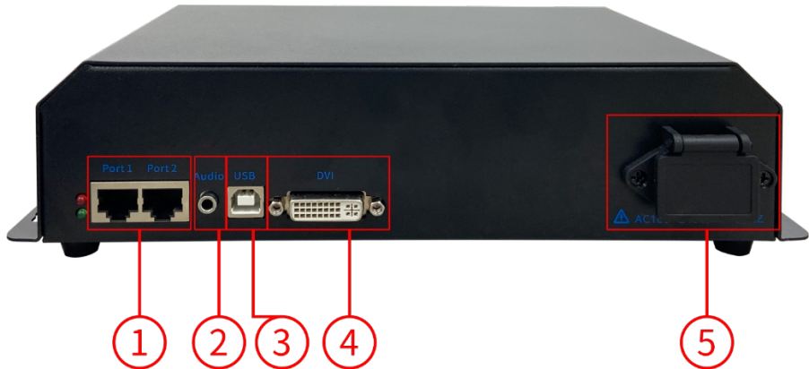
后面板
