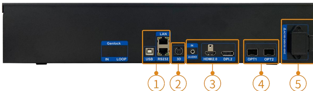
后面板
