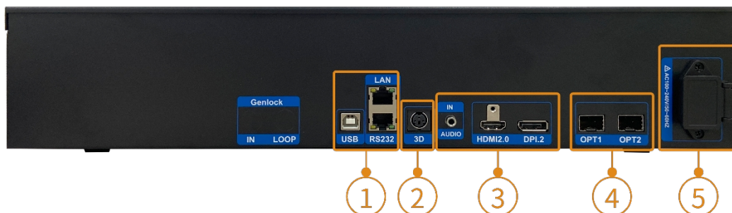
后面板
