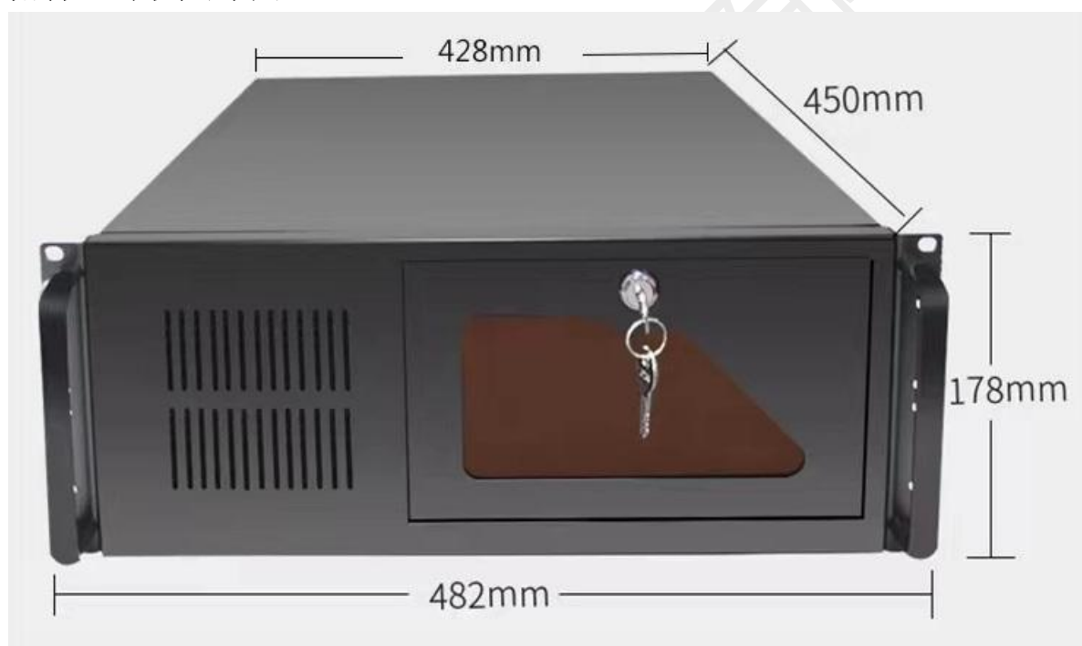
附件：外观尺寸图
