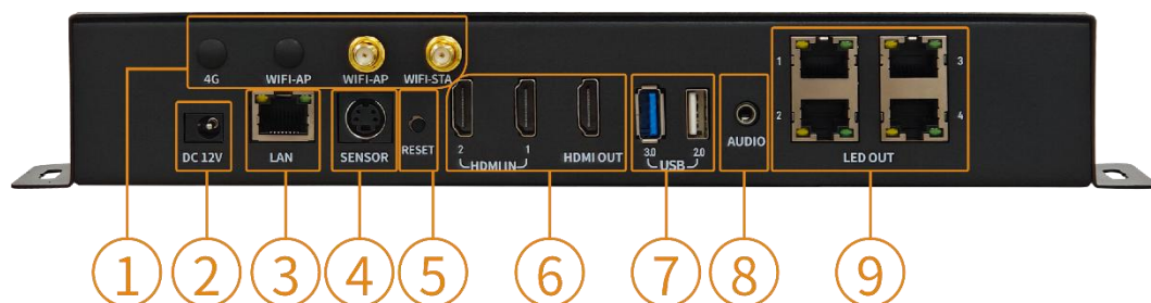
后面板
