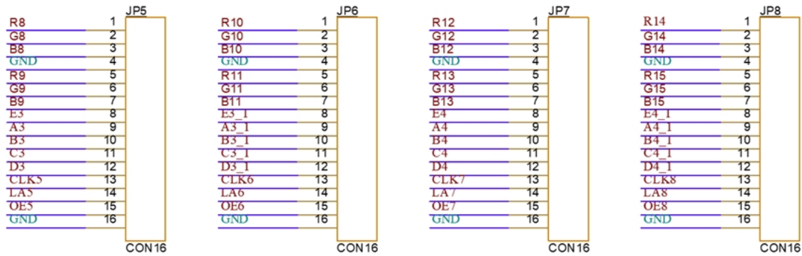
JP1-JP8 数据接口定义
